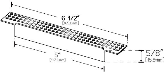
LH16127-EC End Cap
